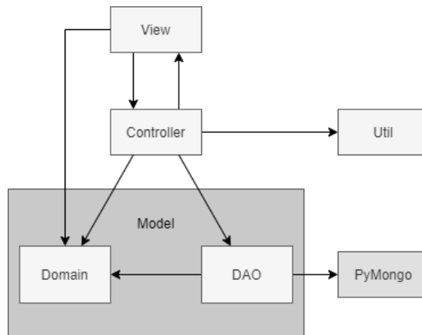
Figura 2.2 – Arquitetura ideal da aplicação PythonToDo
