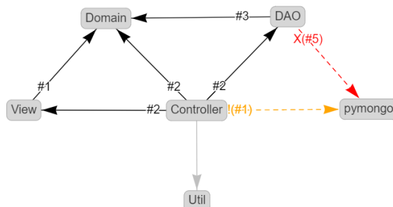
Figura 2.3 – Grafo de reflexão gerado pelo ArchPython
