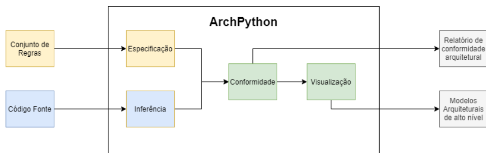
Figura 2.1 – Visão geral do ArchPython
